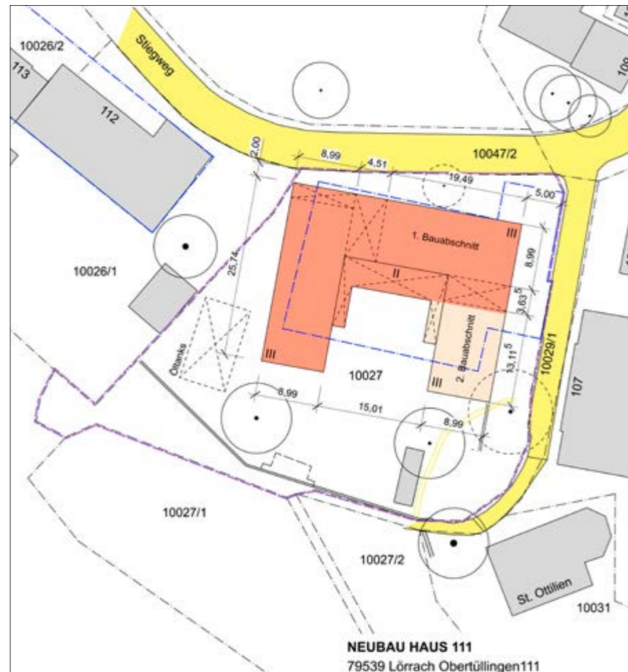
Der Lageplan zeigt die Neuausrichtung des Neubaus nach Süden hin mit der dadurch entstehenden zusammenhängenden Spiel- und Bewegungsfläche
